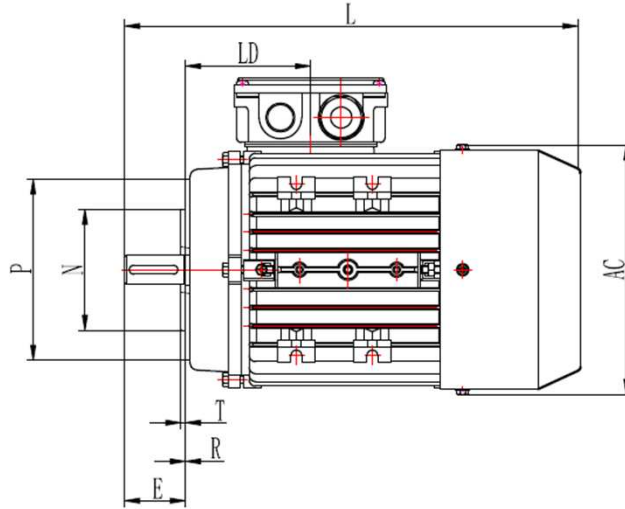
Anbaumaße, mm
